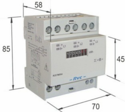
Méreték 70 mm = 4 DIN modul
