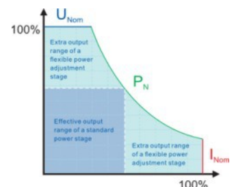
Állandó teljesítmény diagramja
