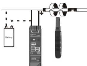
Rövidzár behatárolása
