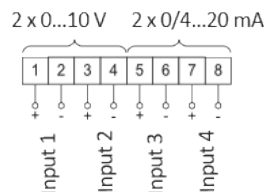
2 feszültség és 2 áram bemenet
