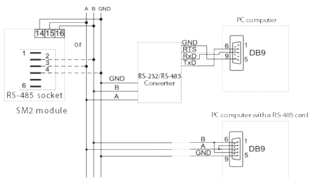
Az RS-485 interfész bekötése
