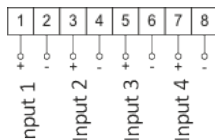
4 feszültség bemenet, 0... 10 V
