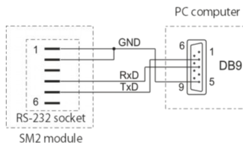
Az RS-232 interfész bekötése
