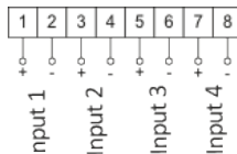
4 áram bemenet, 0/4... 20 mA
